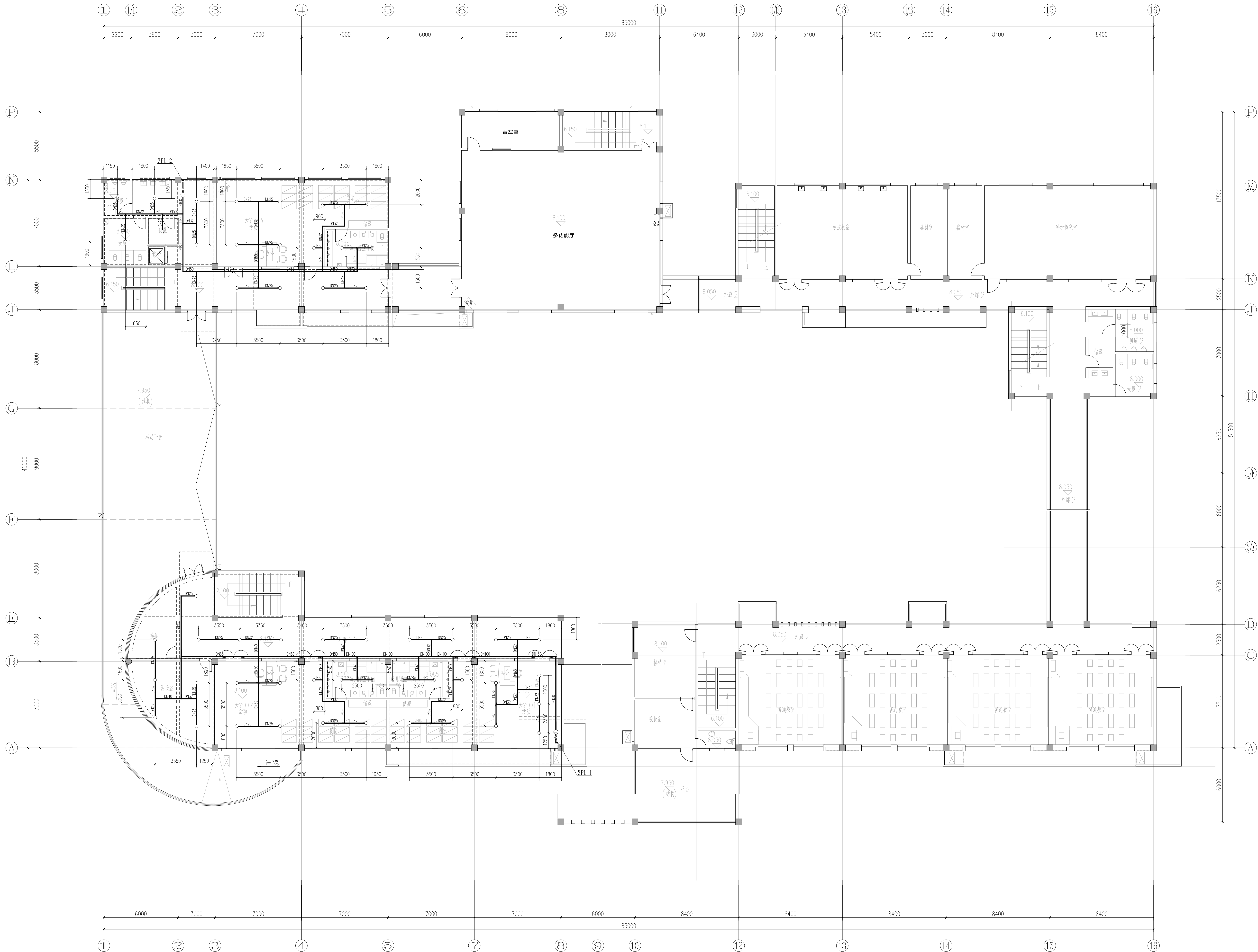
三层喷淋平面图 1:100
